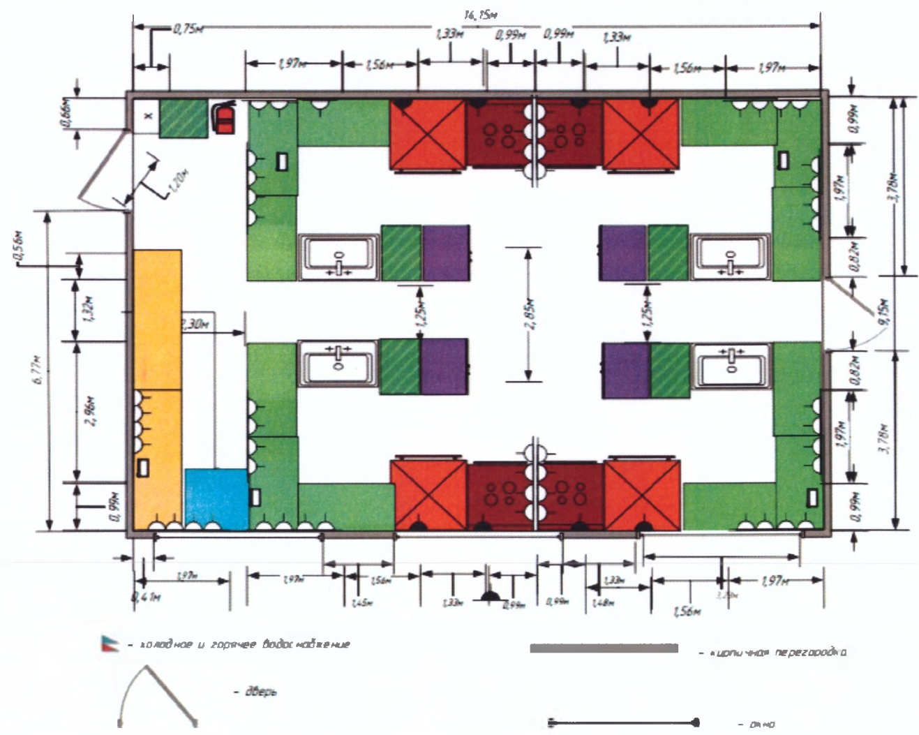
План застройки мастерской по компетенции «Поварское дело» (площадь помещения S=50,64 \text{ м}^2 )
